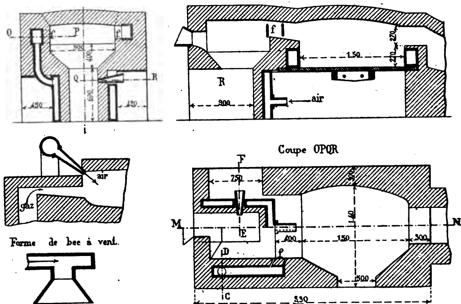
Fig. 98 à 102. — Four de Raisen.
